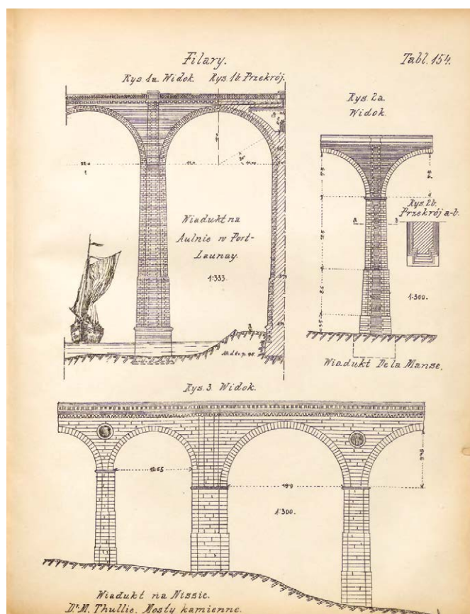
Ilustracja w: Mosty kamienne , Maksymilian Thullie, Lwów 1908. [Politechnika Wrocławska]
