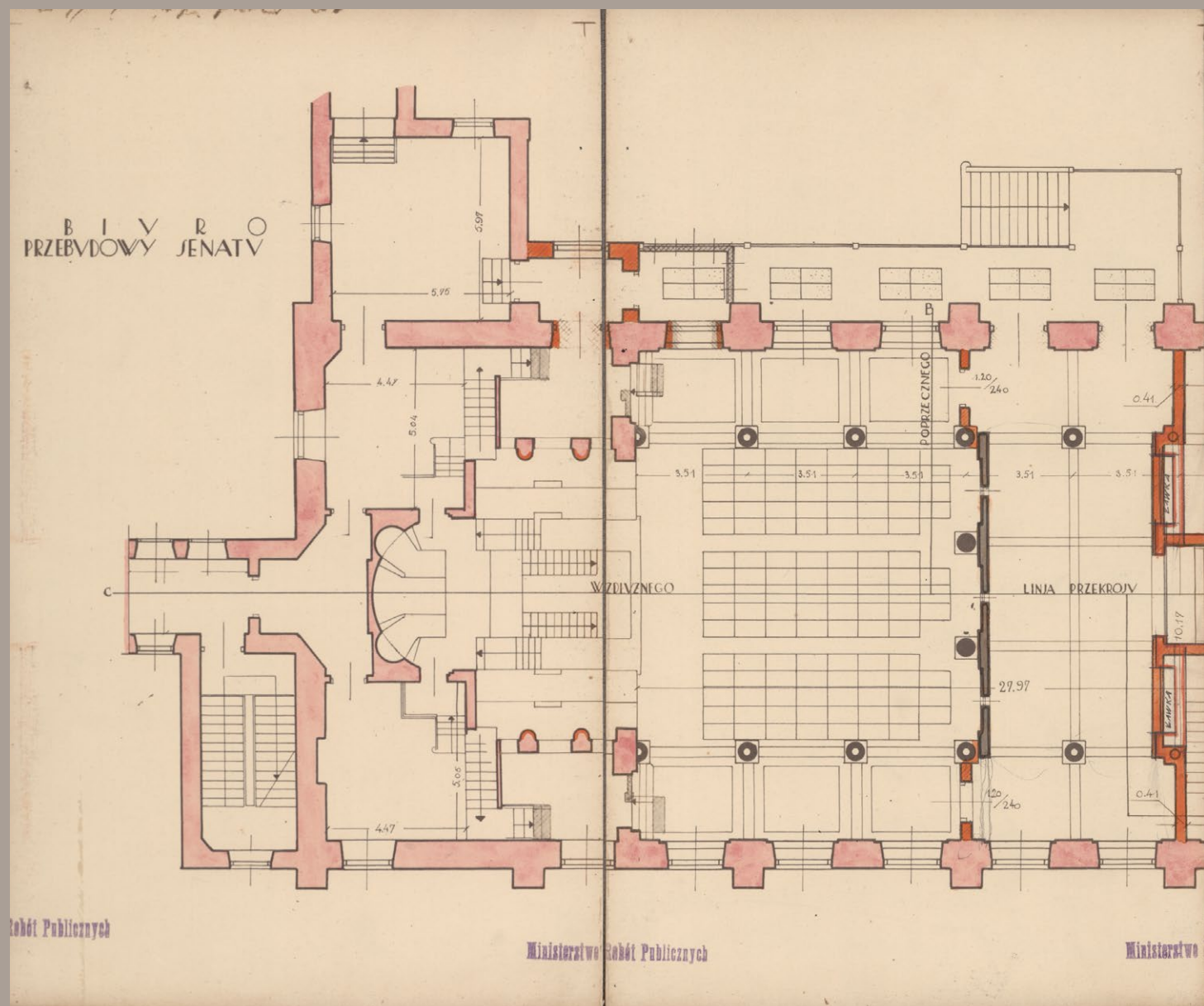
Rzut przyziemia senackiego skrzydła z projektu Stanisława Miecznikowskiego, 1928 r.
