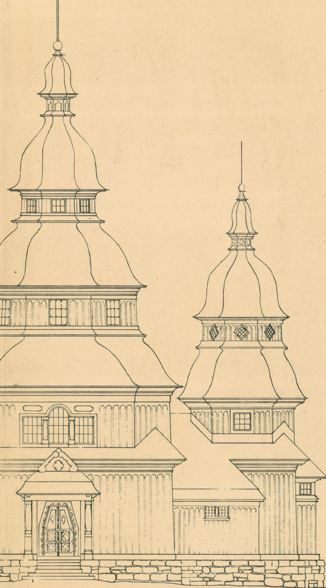
Projekt drewnianej cerkwi we wsi Broniki (pow. Równe) autorstwa senatora Sergiusza Tymoszenki, zatwierdzony przez Ministerstwo Spraw Wewnętrznych w 1923 r.
